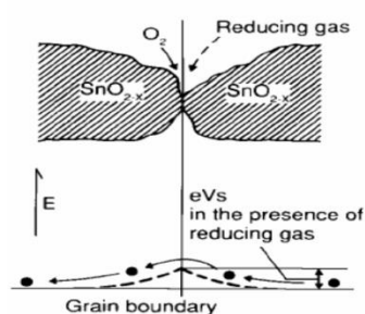
Gambar 12. Model penghalang pada keadaan adanya gas(sumber: Oktorizal,2010)
