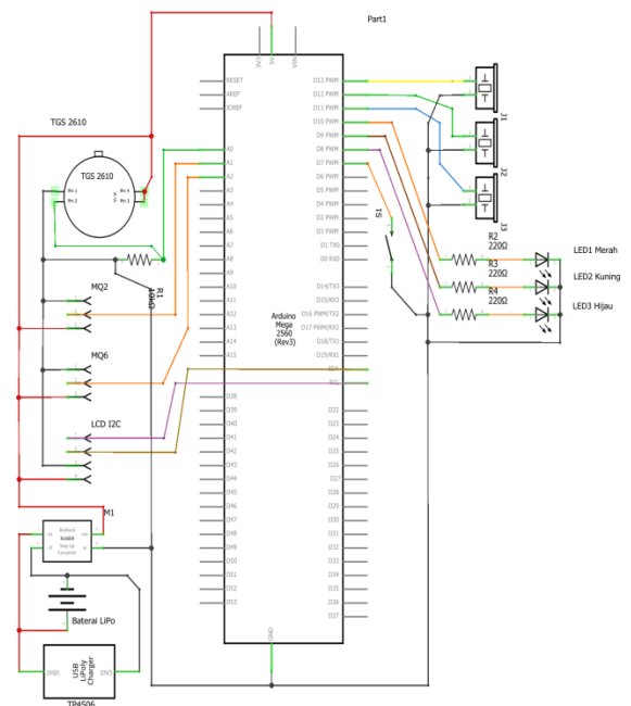
Gambar 4. Skematik rangkaian elektronika alat
