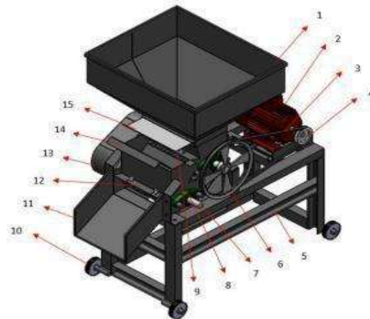
Gambar 1. Desain mesin
