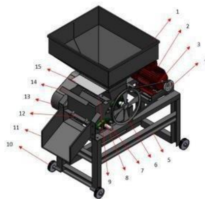
Gambar 2. Desain mesin
