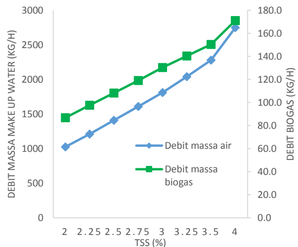
Gambar 6. Debit make up water dan debit biogas terhadap TSS
