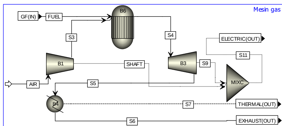
Gambar 4. Mesin gas
