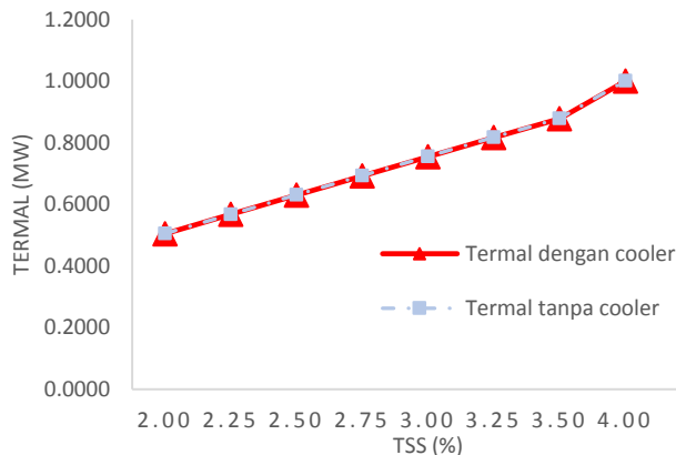
Gambar 10. Daya termal terhadap komposisi TSS
