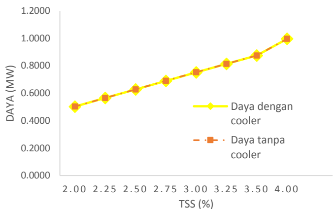
Gambar 9. Daya listrik terhadap komposisi TSS
