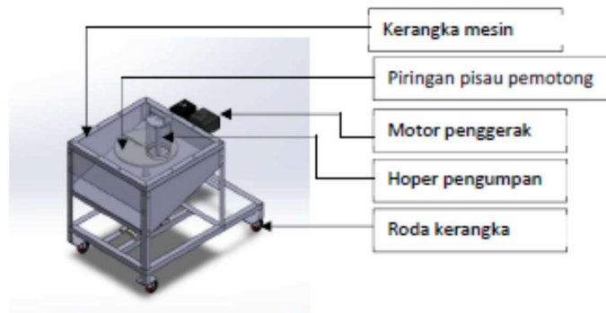
Gambar 2. Rancangan Mesin Pengiris Buah Sukun
