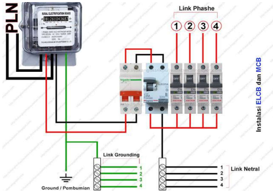
Gambar 2 . Rangkaian instalasi ELCB
